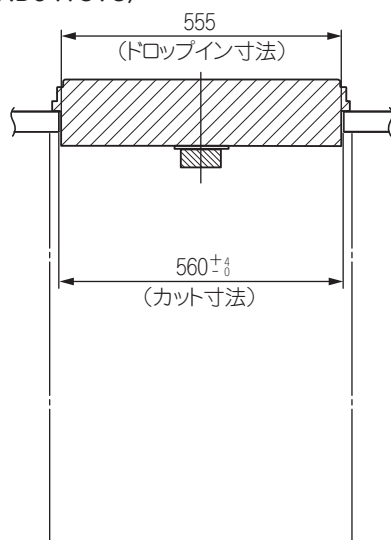
正面図
