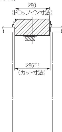
正面図
