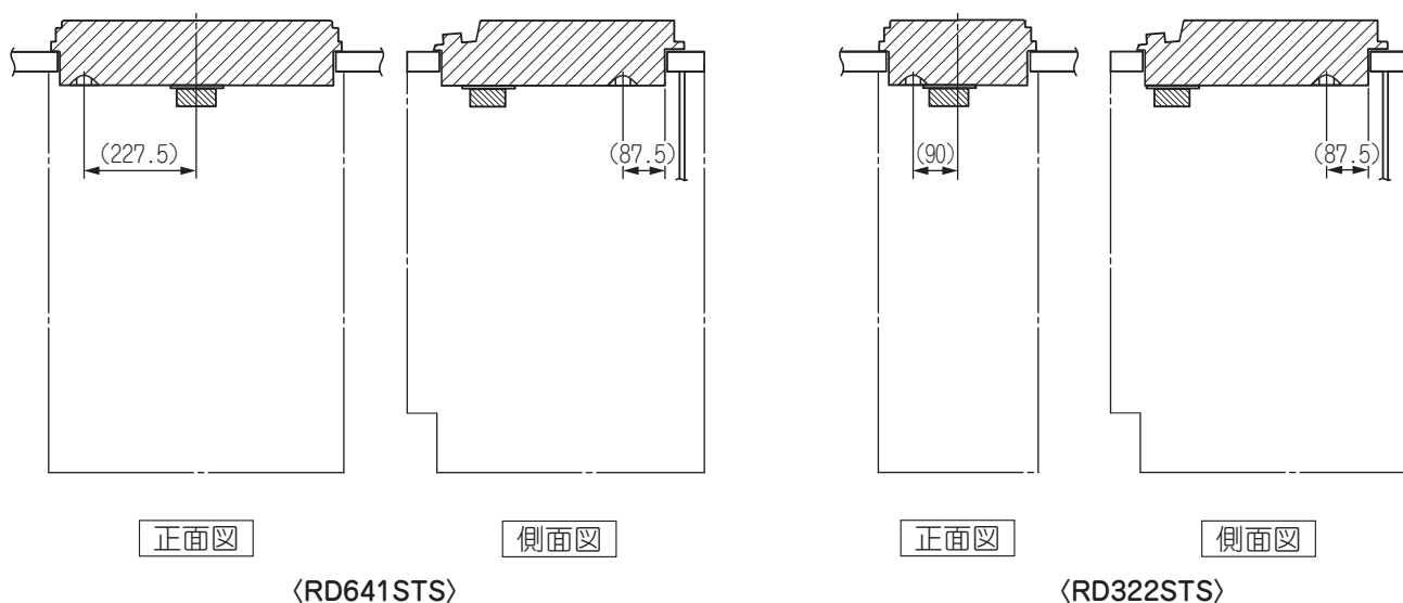
設置施工例図
