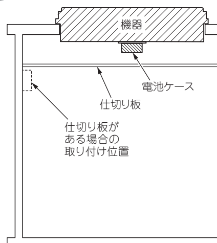
正面図
