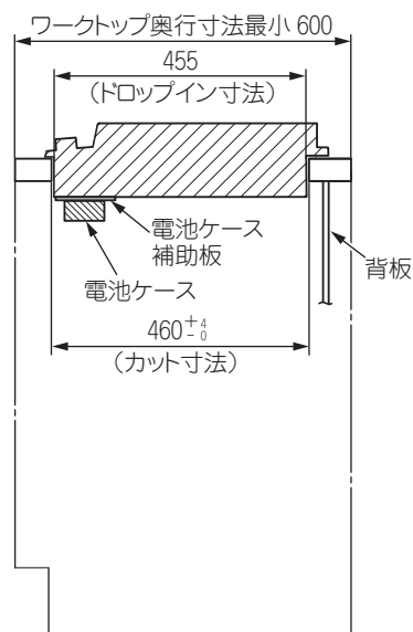
側面図
