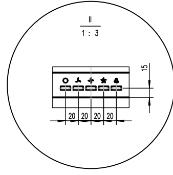
スイッチ部分詳細
