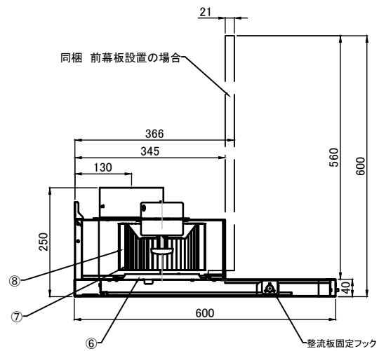
本体取付寸法詳細(左右対称)
