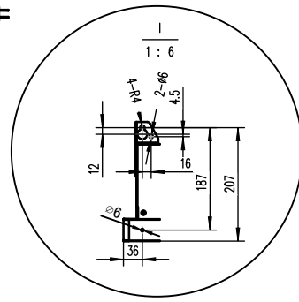
本体取付寸法詳細(左右対称)
